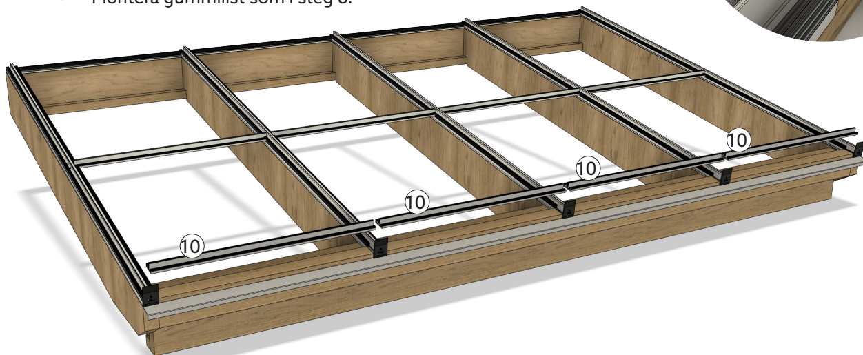
SPRÖJS
