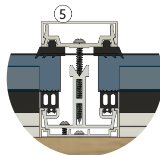
MITTBALK
